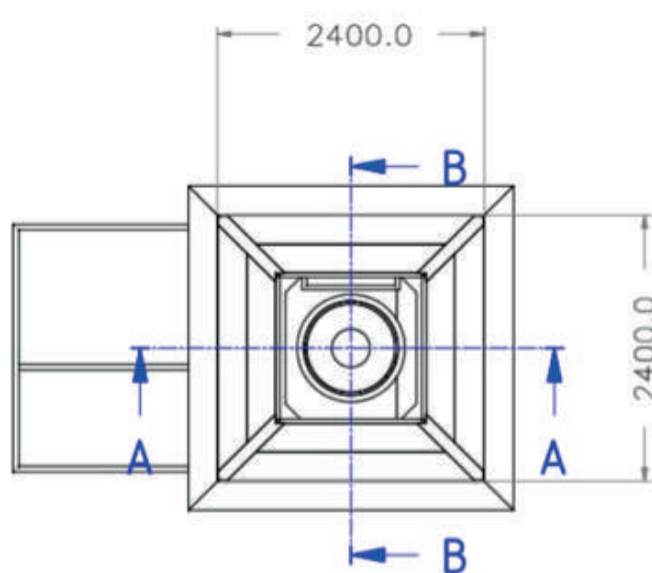
Plano detalle parte superior
